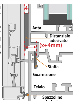
Serramento complanare
