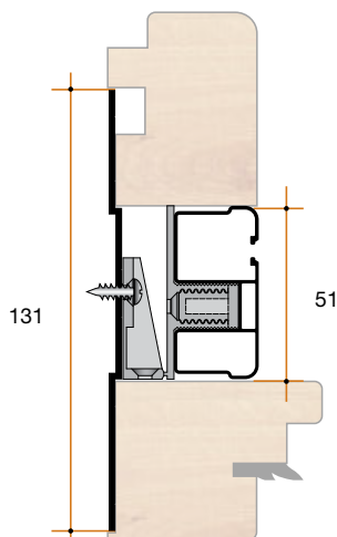
Esempio con guida e compensatore alto
