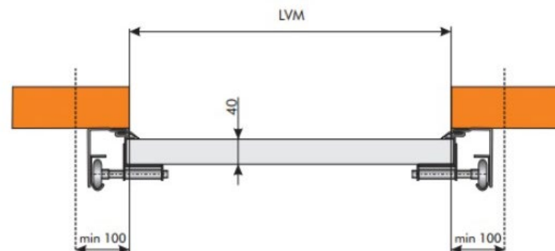
SCHEMA ORIZZONTALE
