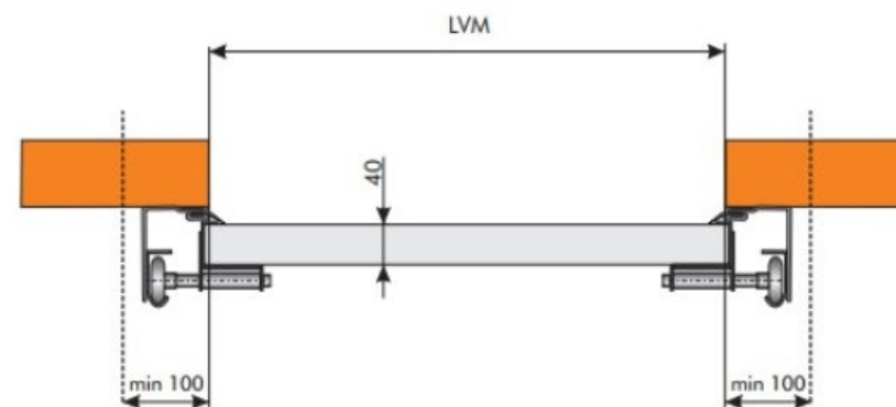
SCHEMA ORIZZONTALE
