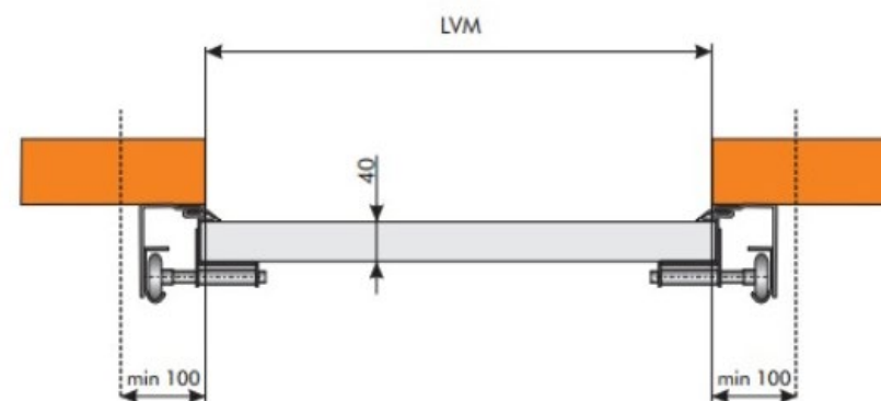
SCHEMA ORIZZONTALE
