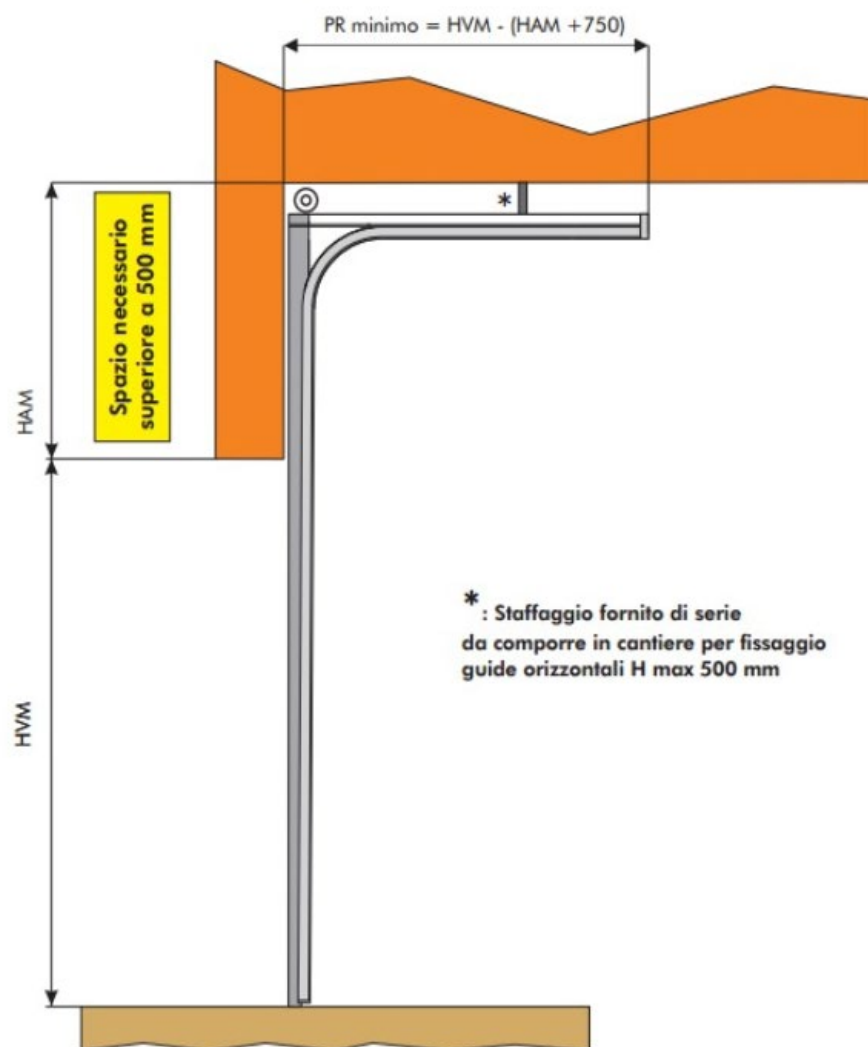
SCHEMA VERTICALE
